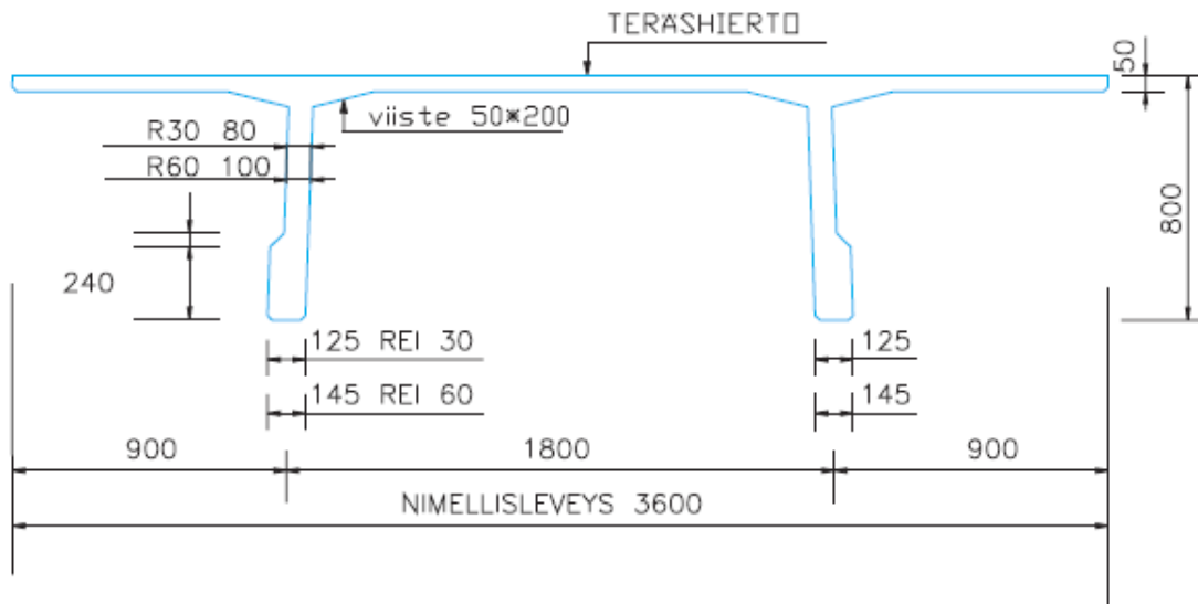
KUVA 1 TTK ( "KovaTT" ) -laattojen poikkileikkausmitat
